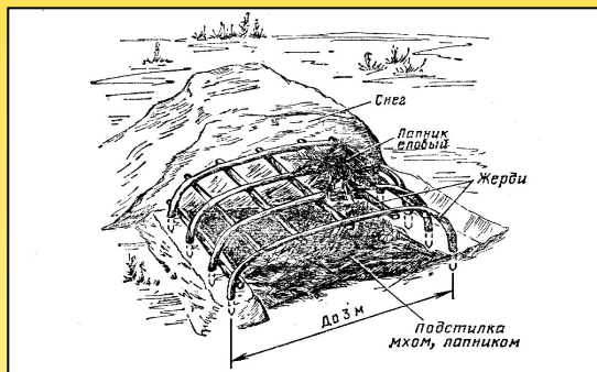
Курінь зі сніжних валів із жердяним покриттям
