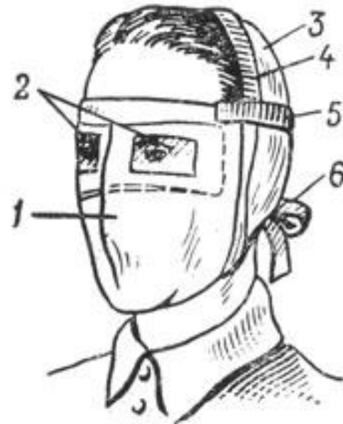
Противопыльная тканевая маска ПТМ-1.
