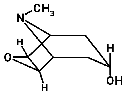
скопин
