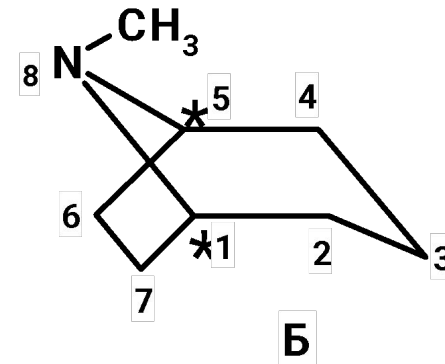
Тропан
