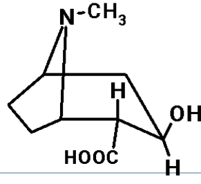
-OH -цис -COOH -транс
