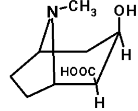
-OH -цис -COOH -цис
