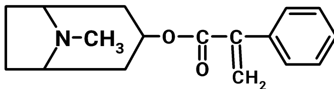
апоатропин
