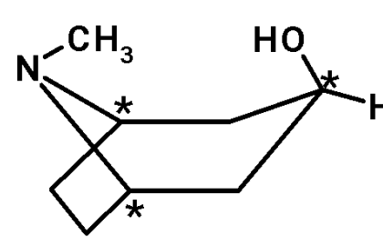
Псевдотропин (цис-изомер)
