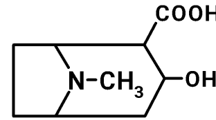
экгонин (тропин-2-карбоновая кислота)
