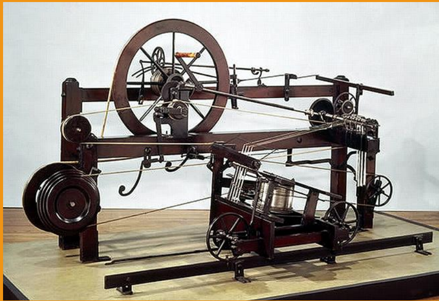
Прядильная машина 1774 г.
