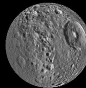
Mimas
