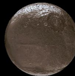
Iapetus
