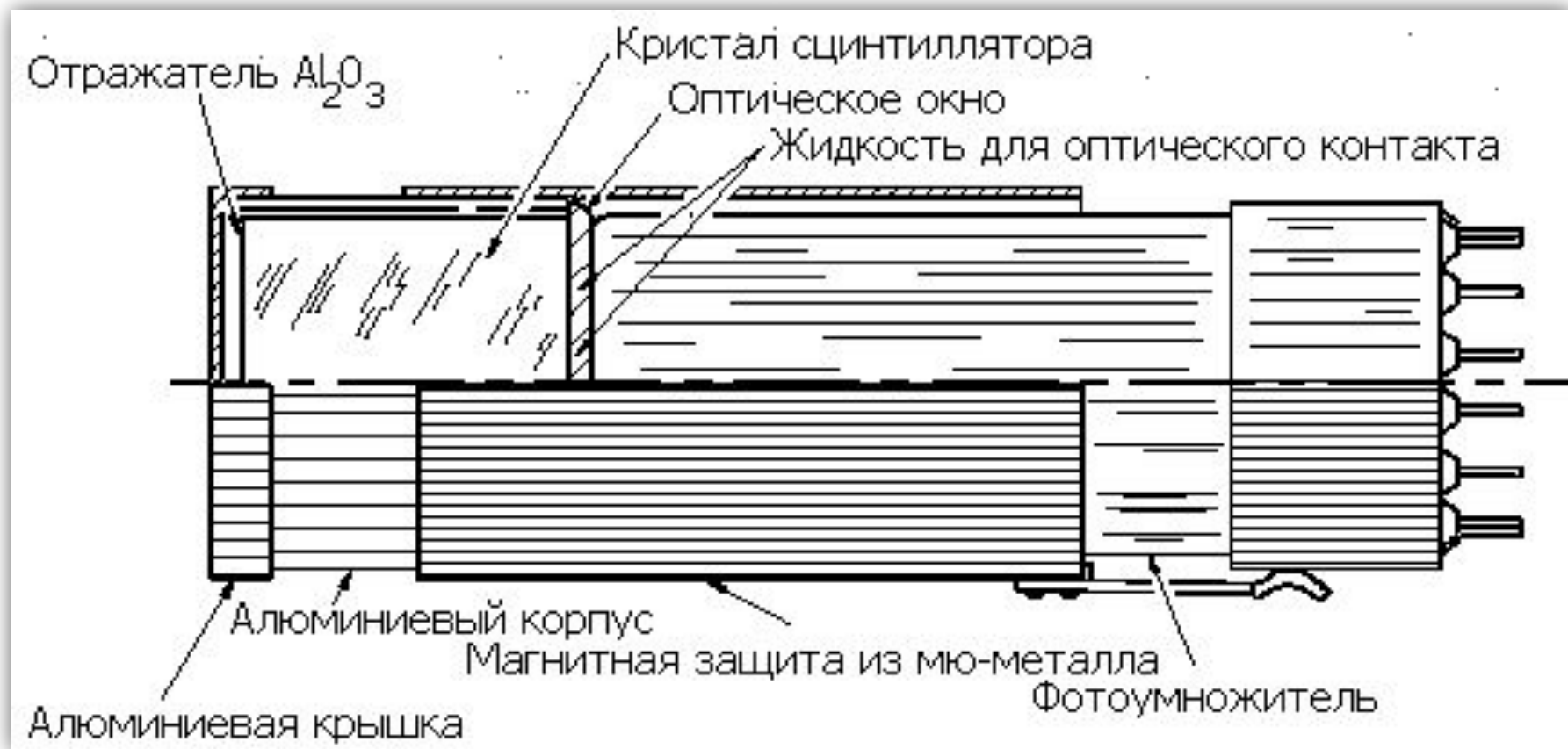
Сцинтиллятор и ФЭУ
