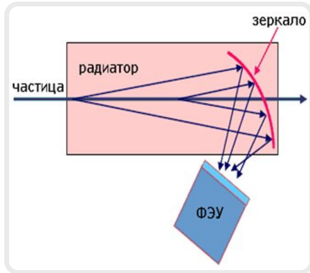
Схема порогового счетчика
