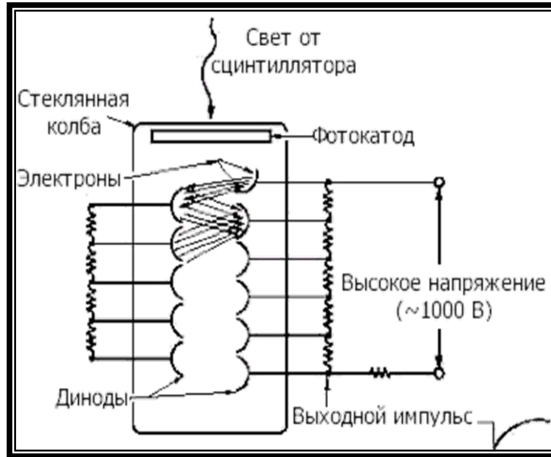
Устройство ФЭУ
