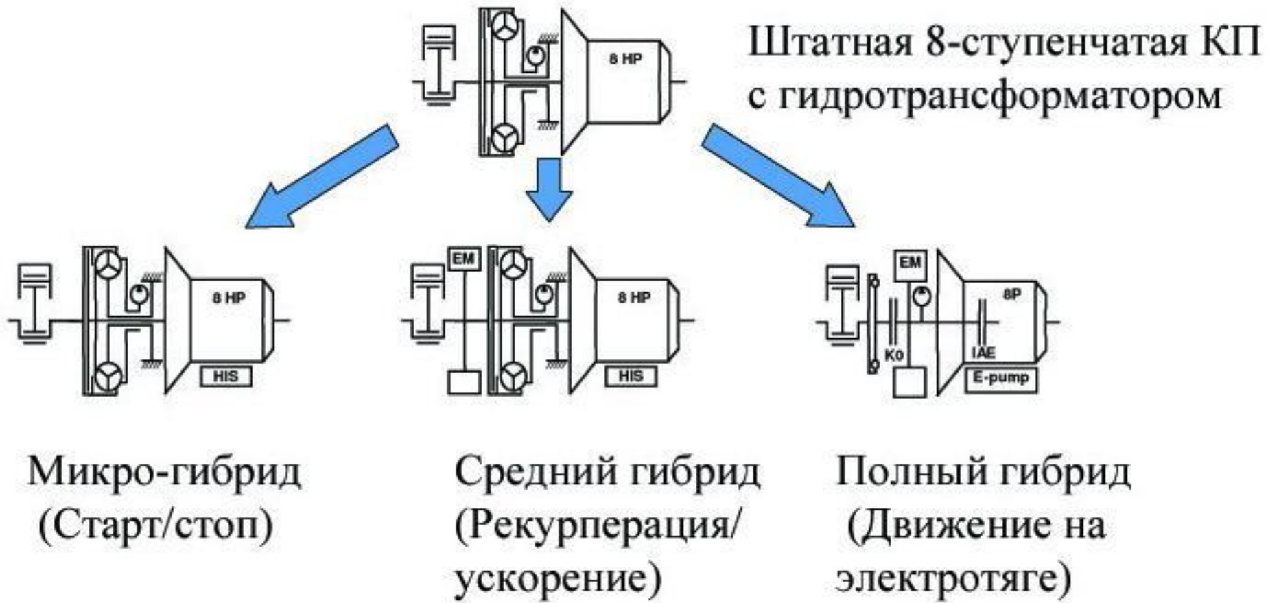
Рисунок 3 - параллельные гибридные трансмиссии
