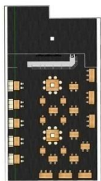
План с экспликацией мебели
