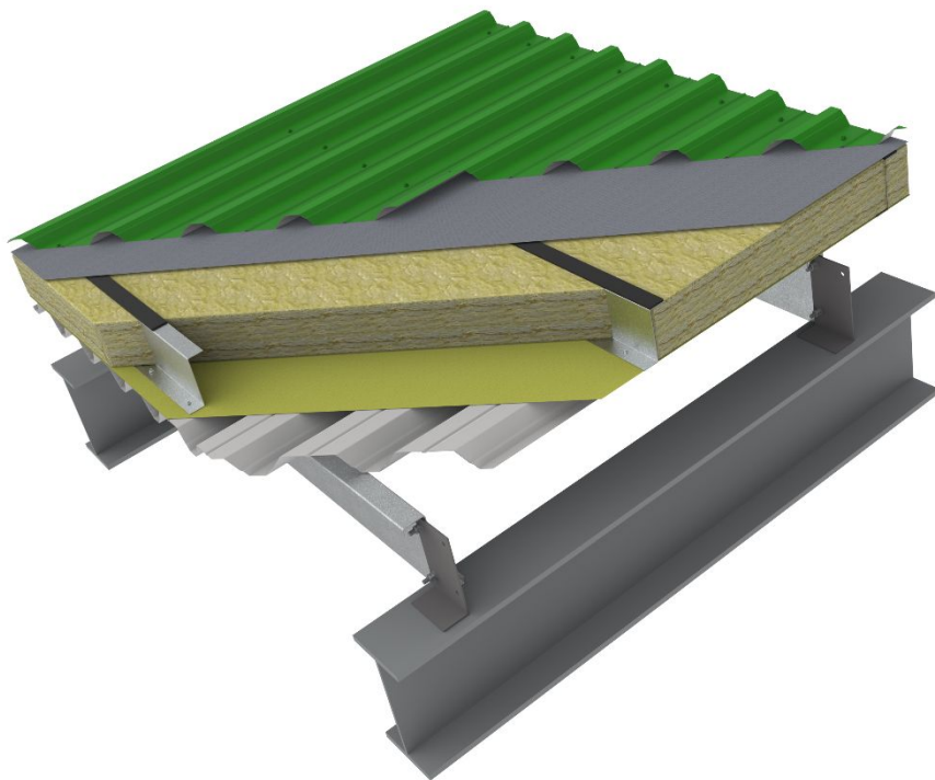
Конструкція «теплої» покрівлі прогонна
