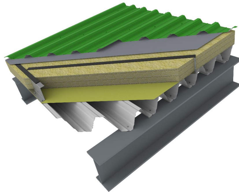
Конструкція «теплої» покрівлі безпрогонна
