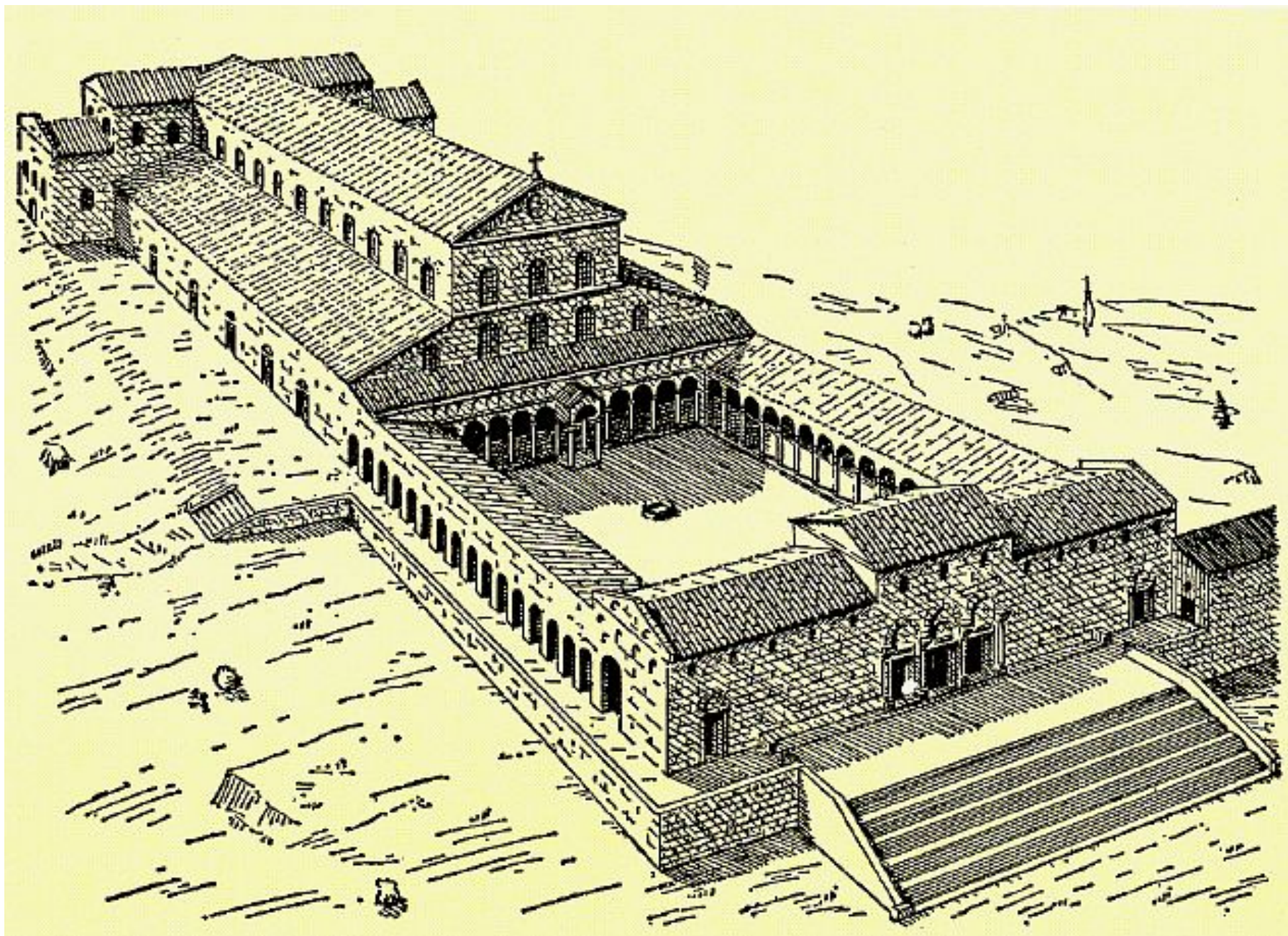
Базилика Св. Петра. Реконструкция. 4 в. Рим.
