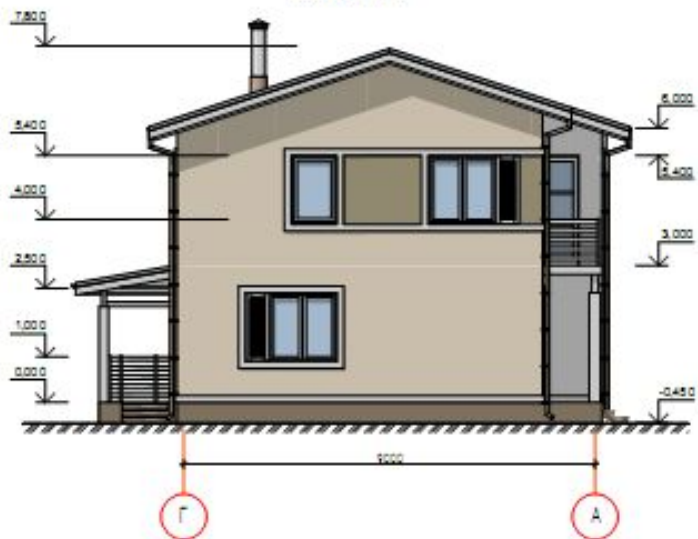
Фасад Г - А
