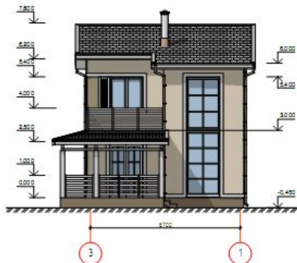
Фасад 3 - 1
