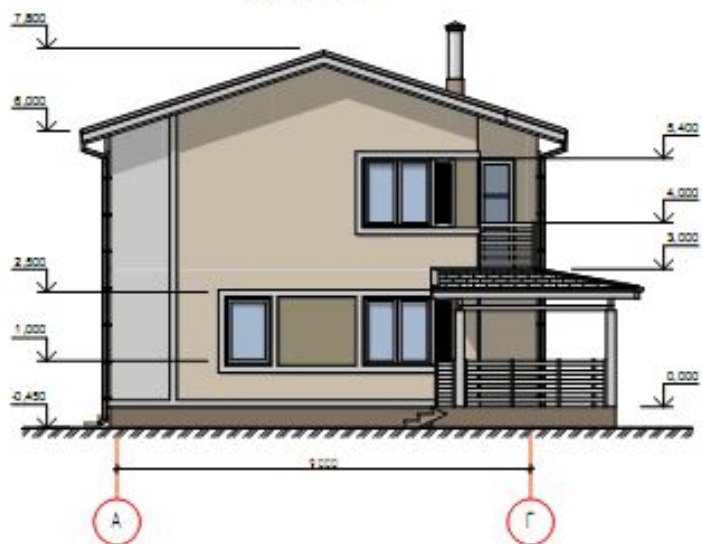
Фасад А - Г
