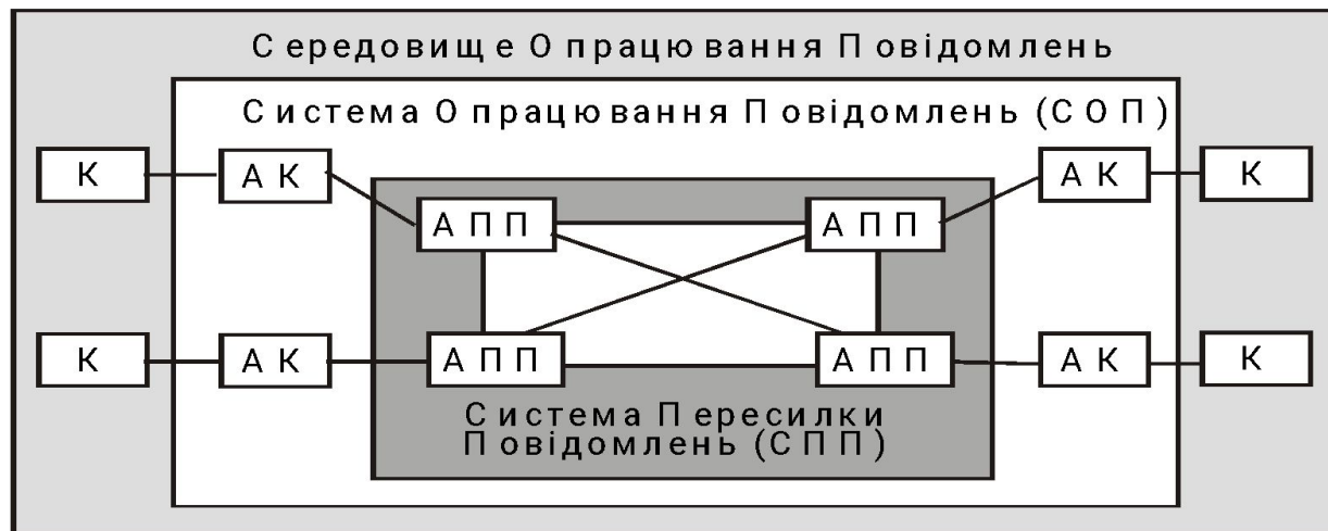
Модель системи Опрацювання повідомлень відповідно до рекомендацій МККТТ Х.400 (1984 р.)
