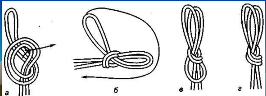
Рис. 63. «Двойной проводник»
