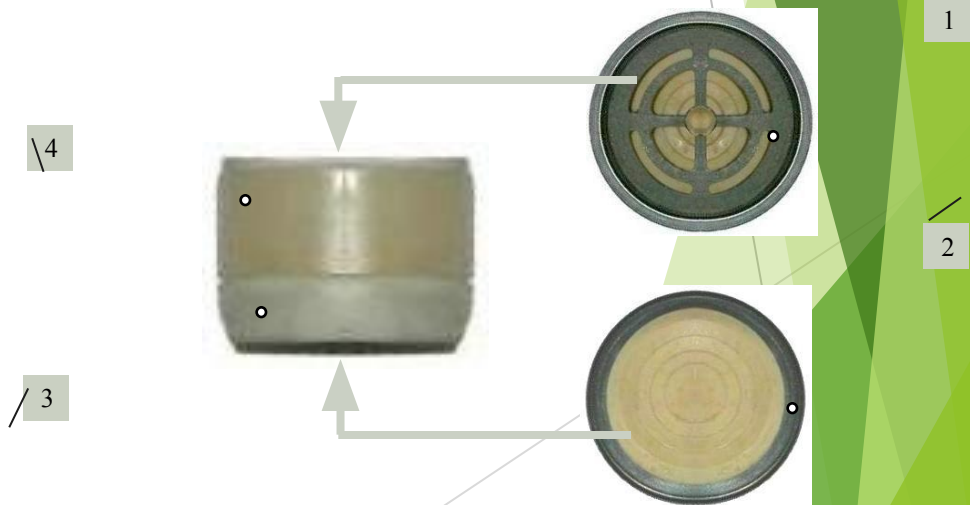
Клапанная коробка противогаза ПМГ: 1 - клапан выдоха (внутренний); 2 - клапан выдоха (наружный); 3 - патрубок выдоха; 4 - втулка монтажная.
