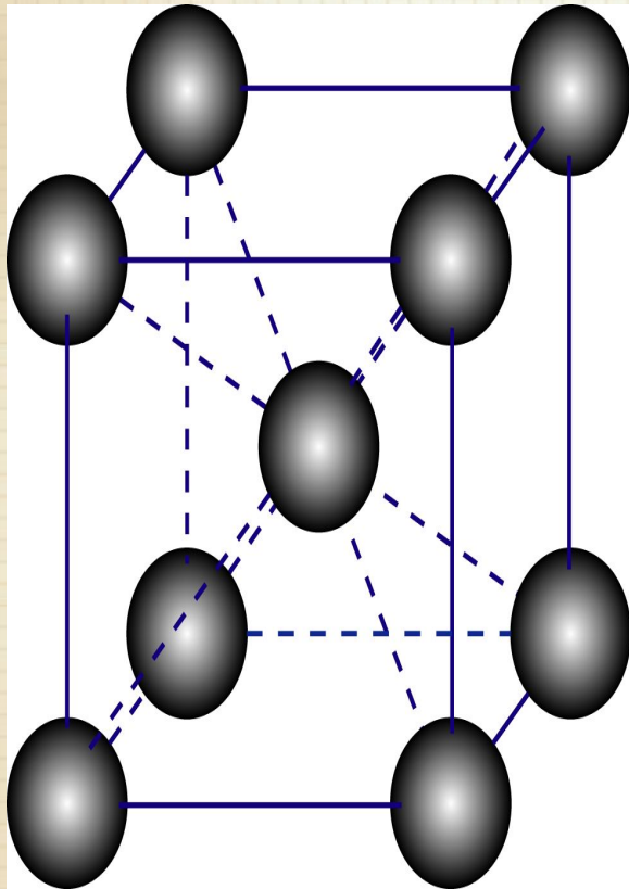
Кубическая объёмноцентрированная
