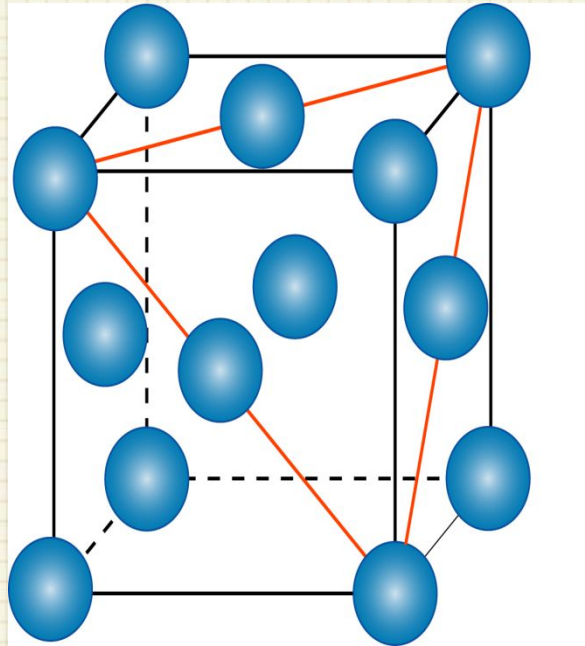
Кубическая гранецентрированная
