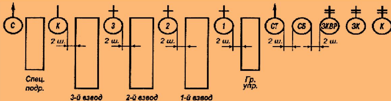
Рис. 13. Развернутый строй роты - в линию взводных колонн
