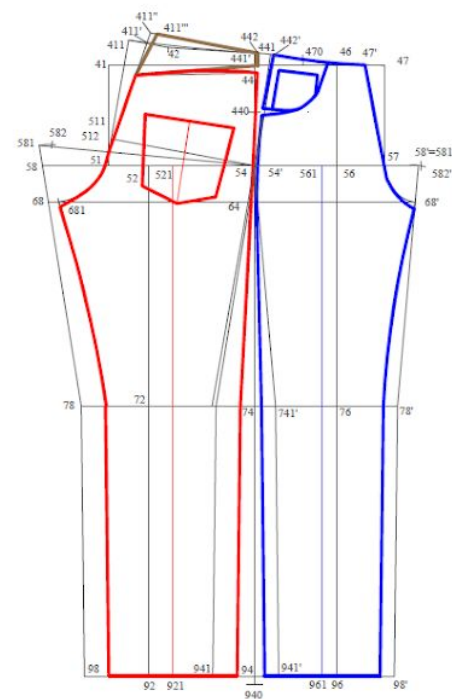
Рисунок 5.24 — МК классических джинсов
