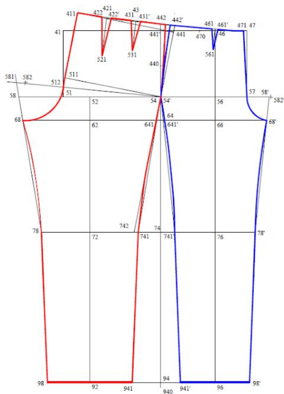
Рисунок 5.10 — ИМК женских брюк
