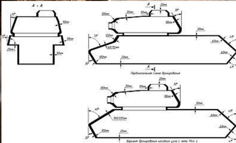
Схема бронирования танка ИС-2
