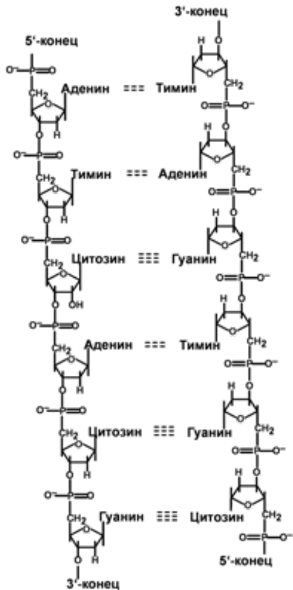
Строение ДНК
