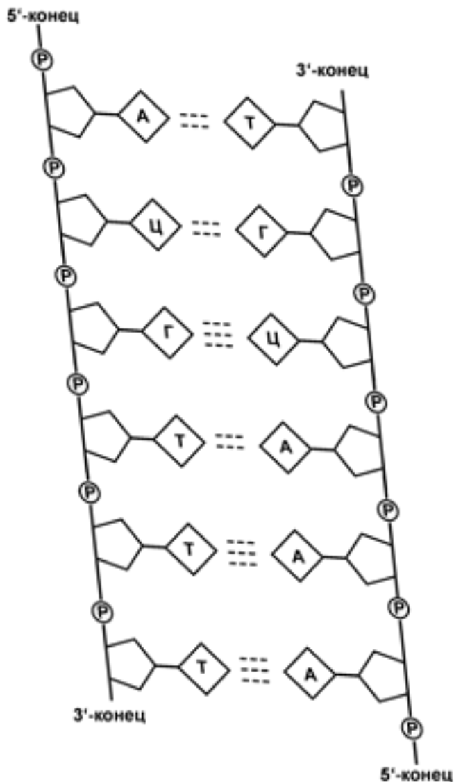
Схематичное строение ДНК
