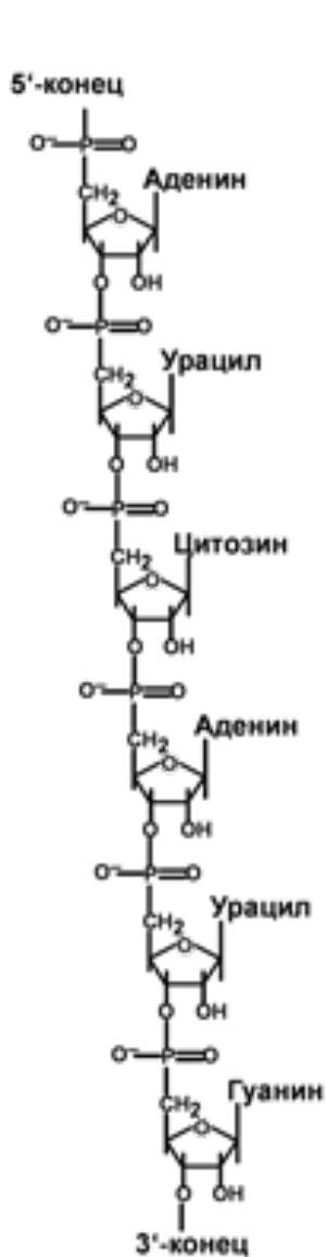
Строение РНК
