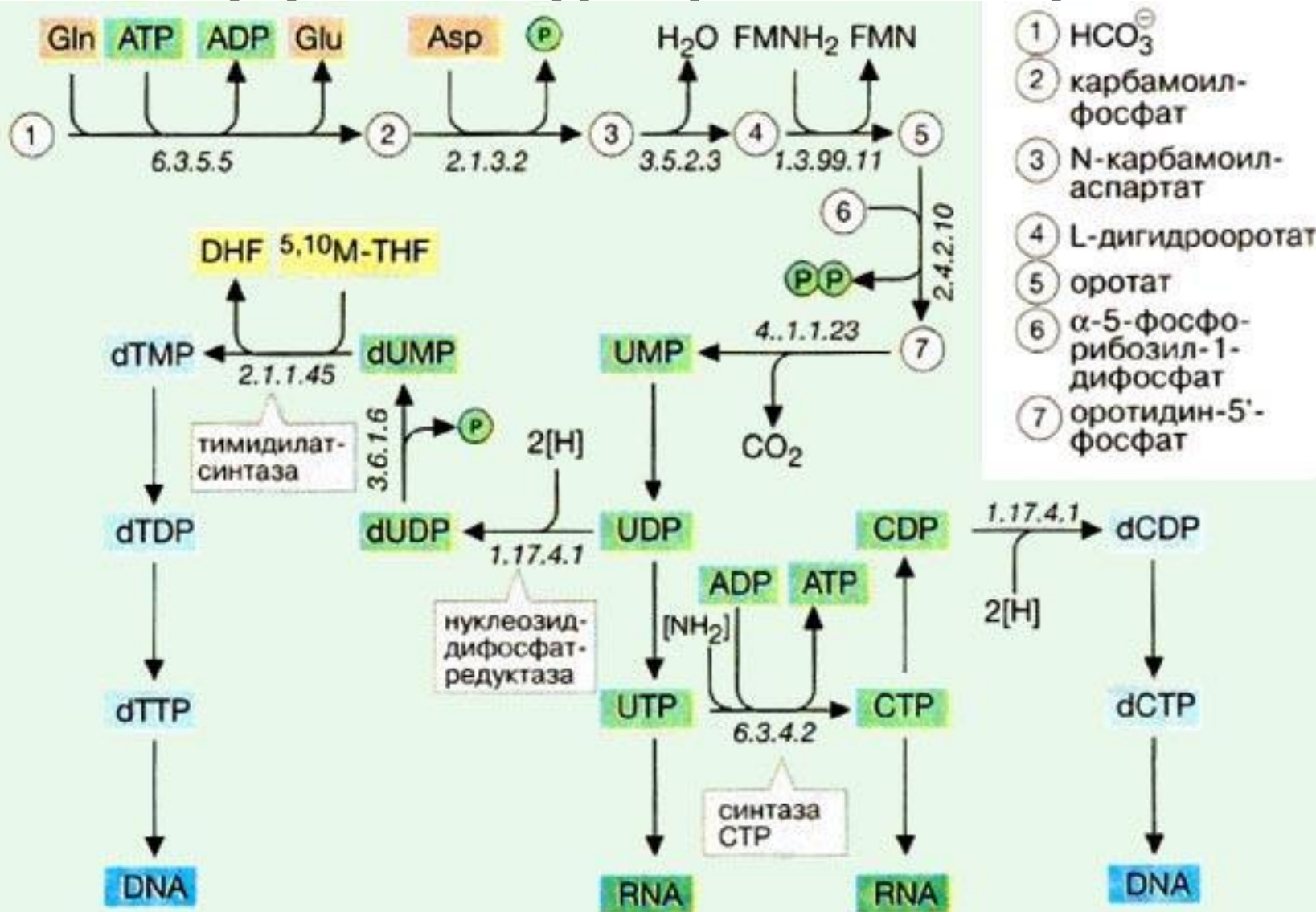
А. Биосинтез пиримидиновых нуклеотидов
