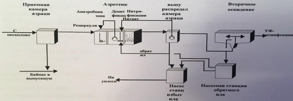
Рис 1. Процесс активного ила.
