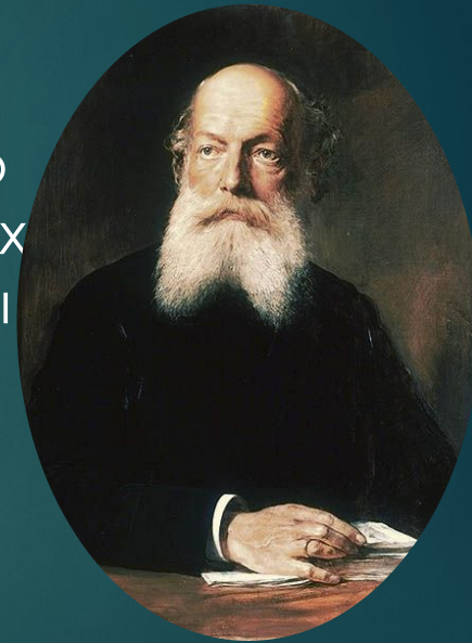
Фридрих Кекуле
