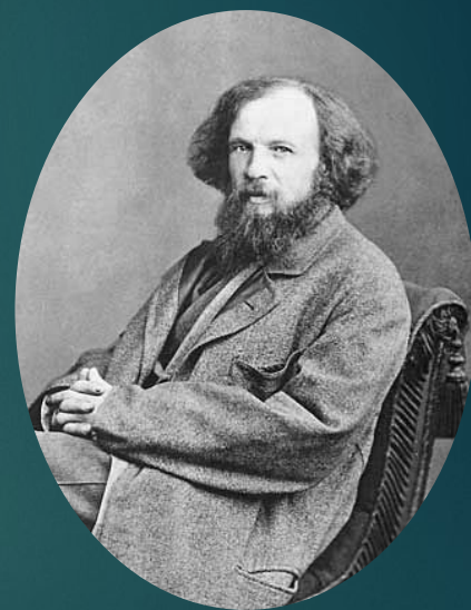
Дмитрий Менделеев
