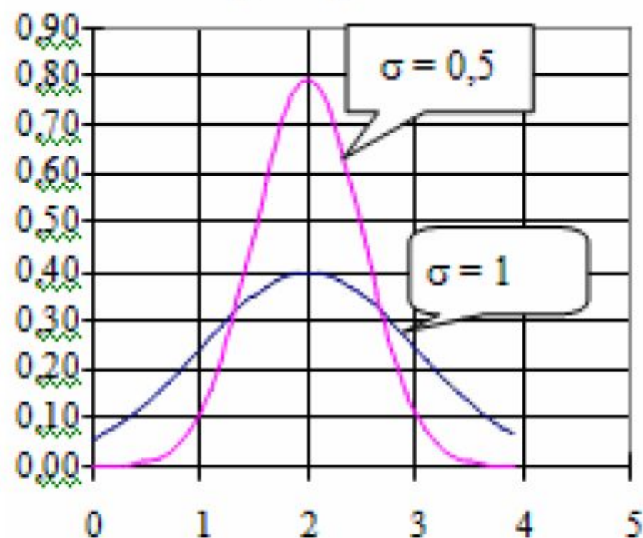
Плотность нормального распределения
