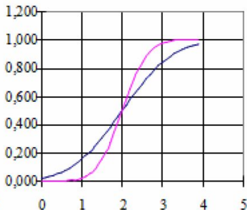
Функция нормального распределения
