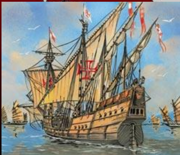
Португальская каравелла
