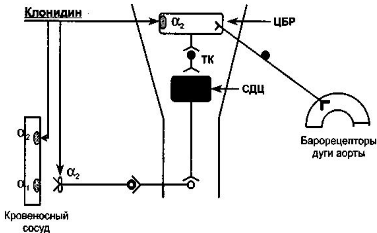
Рис. 45. Механизм влияния клонидина на кровеносные сосуды.
