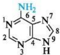
аденин Ade
