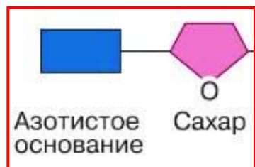
аденин Ade
