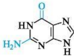
гуанин Gua
