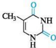
тимин Thy
