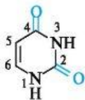
урацил Ura
