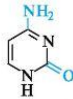
цитозин Cyt
