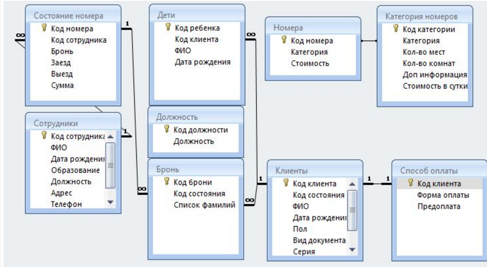
Рисунок 5 – Схема данных
