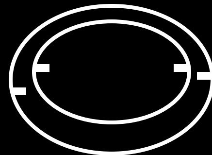
мульда
