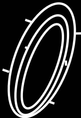
брахиморфная
