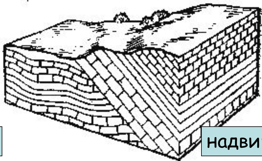
сдвиг
