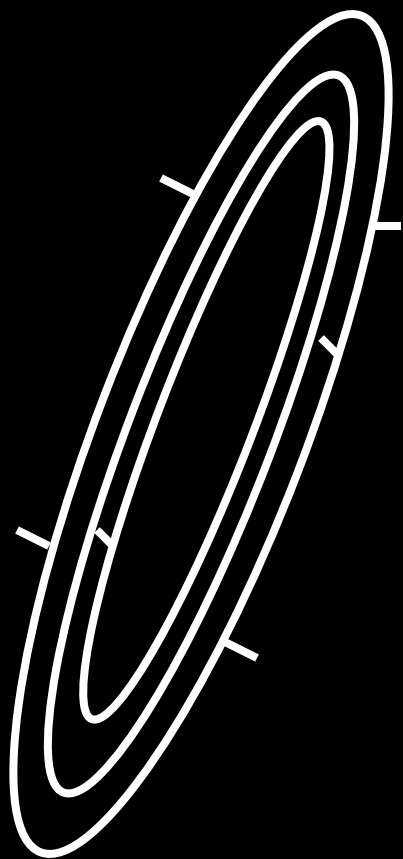
линейная
