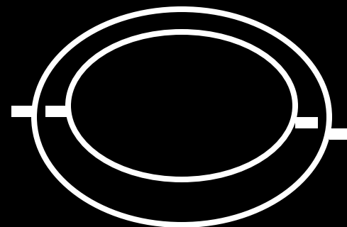
куполовидная
