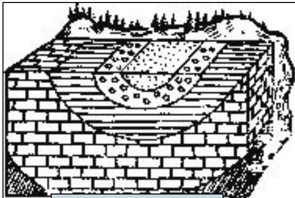
синклиналь
