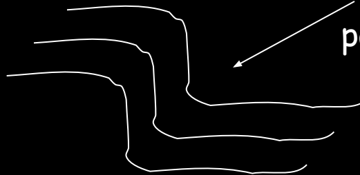
флексура
