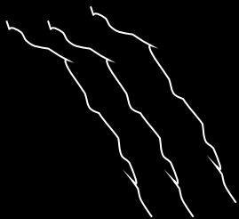
МОНОКЛИНАЛЬ
