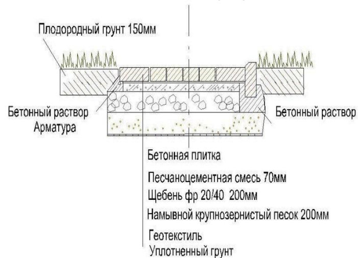
Схема мощения дорог из бетонной плитки в разрезе.
