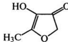
2-Н-4-гидрокси- 5-метилфуранон-3
