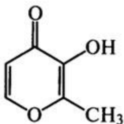
мальтол
