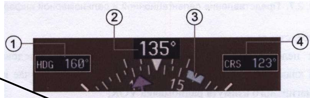
Рис. 3.9. Индикация значений заданного курса (HDG) и ЗПУ (CRS)
