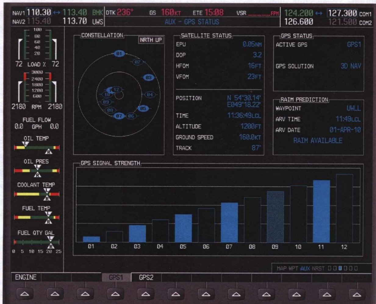
Рис.3.3.2. Третья страница “GPS STATUS” группы AUX на MFD
