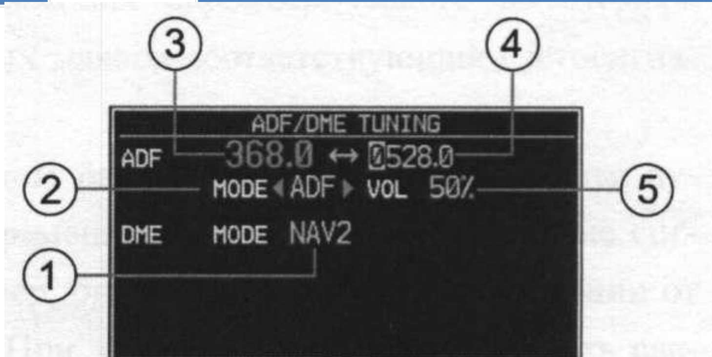
Рис. 3.16. Информационное окно для настройки АРК и дальномера DME
