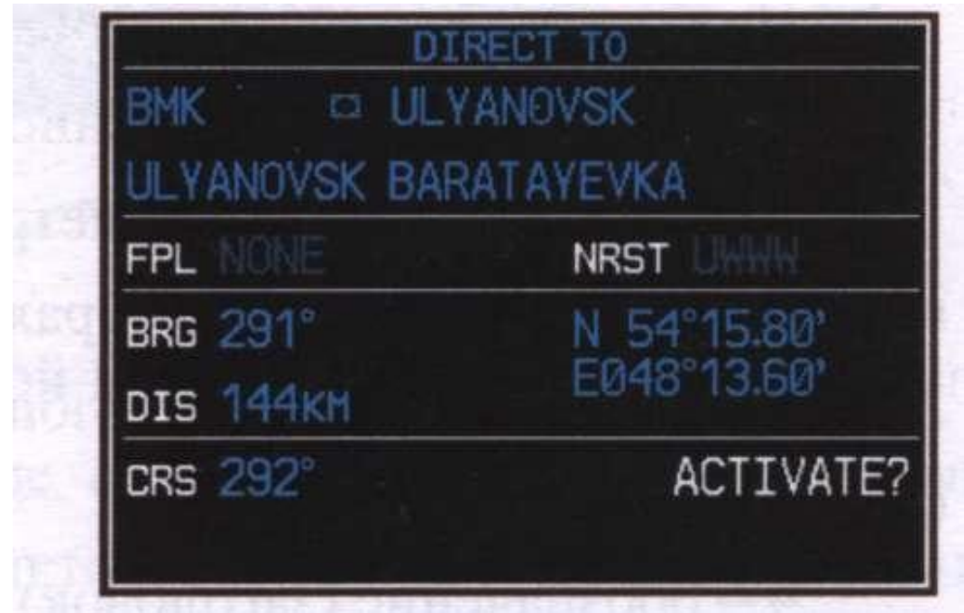
Рис.3.3.9. Диалоговое окно режима «DIRECT TO» на дисплее PFD
