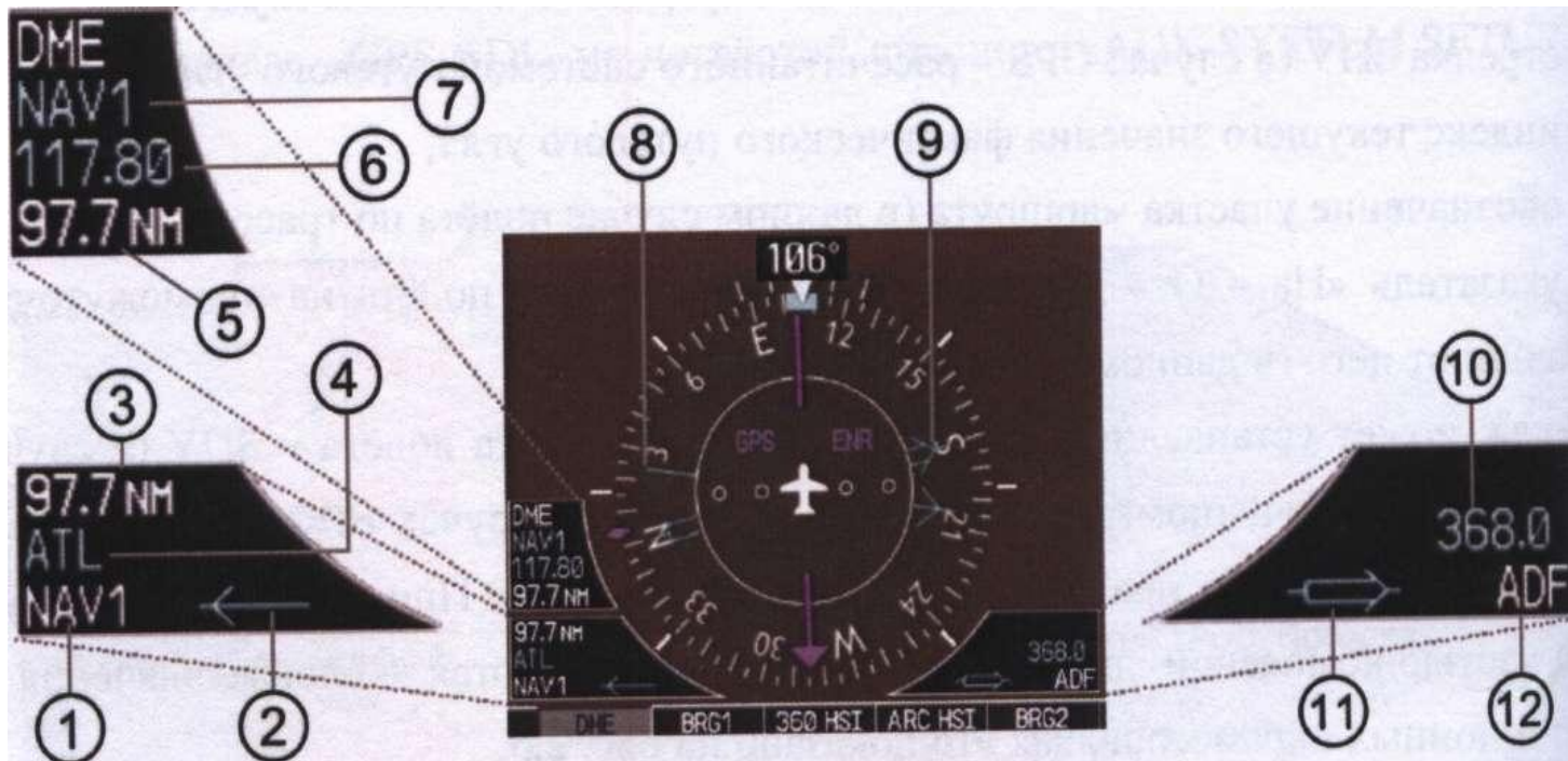
Рис. 3.11. Представление пеленгационной и дальномерной информации
