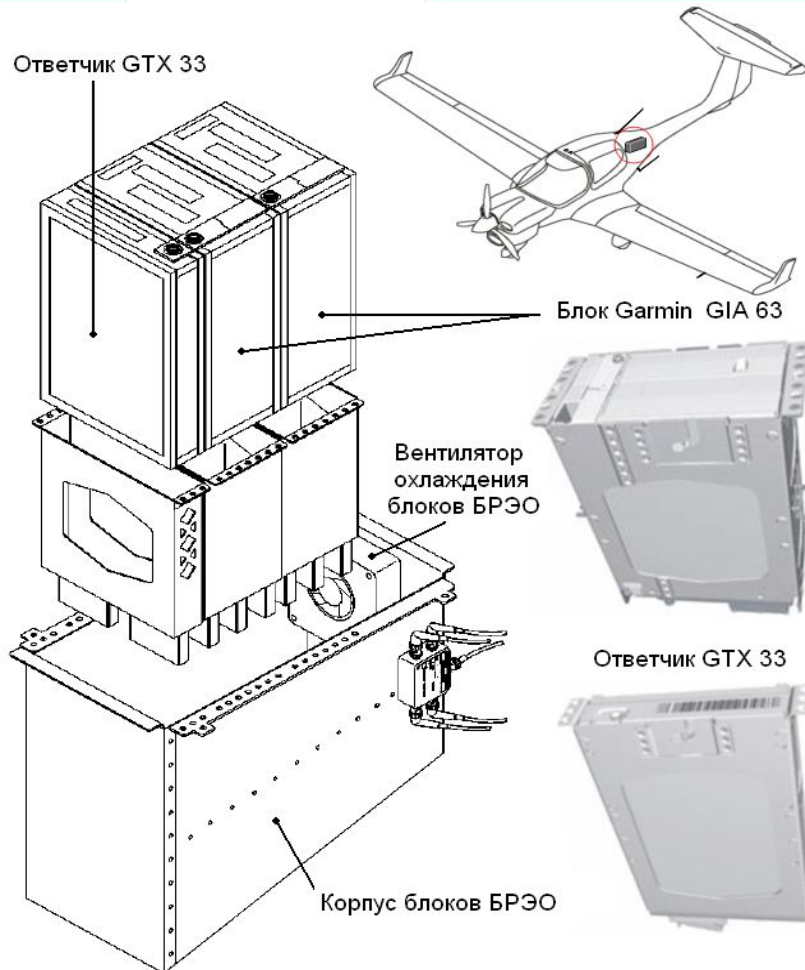
Рис. 4.1.1. (GIA 63, ответчик GTX 33, АРК и курсовертикаль под задним багажным отсеком)
