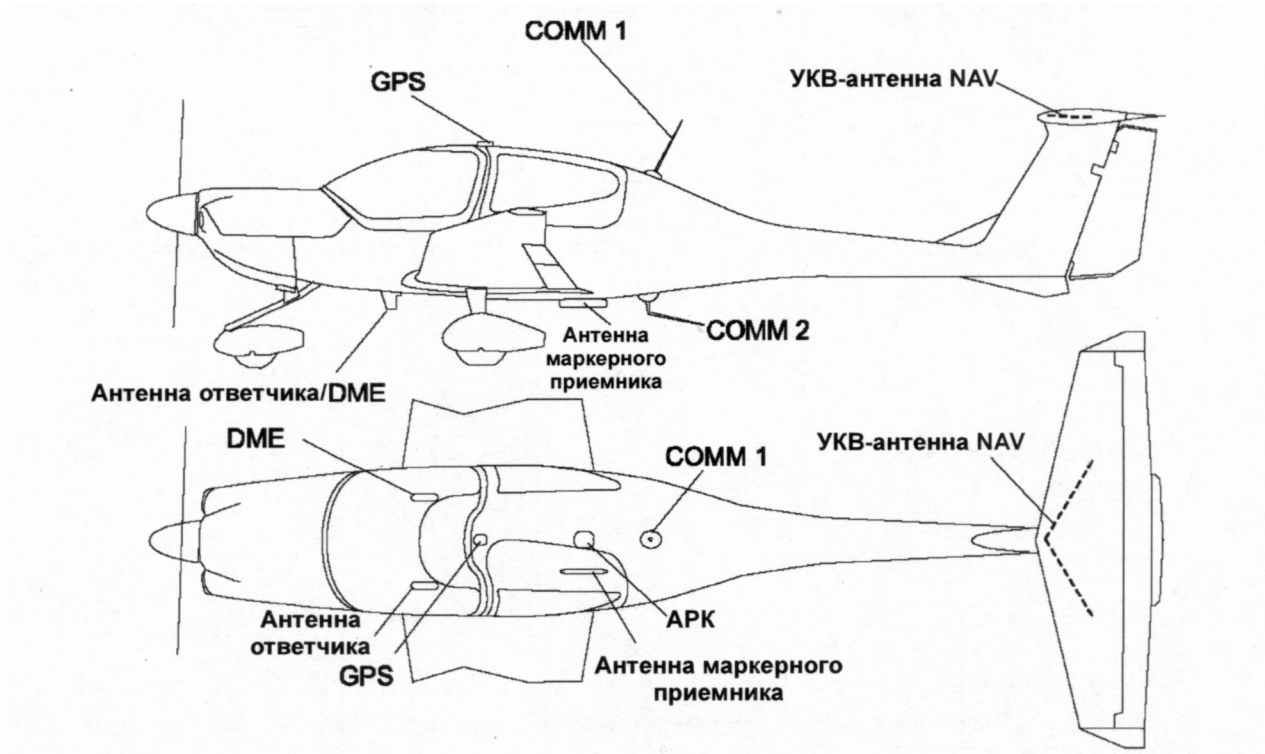
Рис. 3.1 Размещение радиосвязных и радионавигационных антенн
