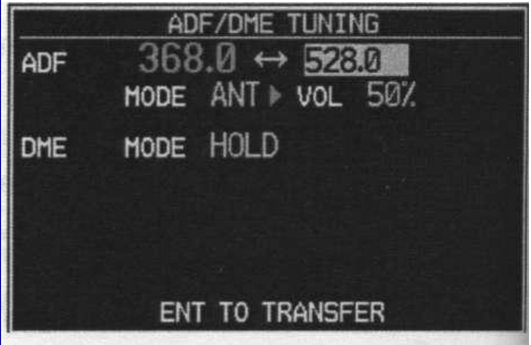
Рис.3.17. Перемещение рабочей и подготовленной частот
