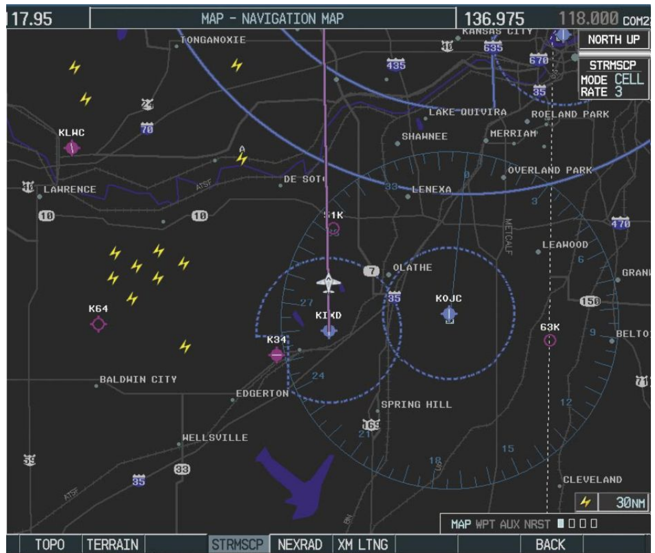
Рис. 2.25. Отображение отметок молний на экране дисплея MFD в совмещённом режиме на странице NAVIGATION MAP
