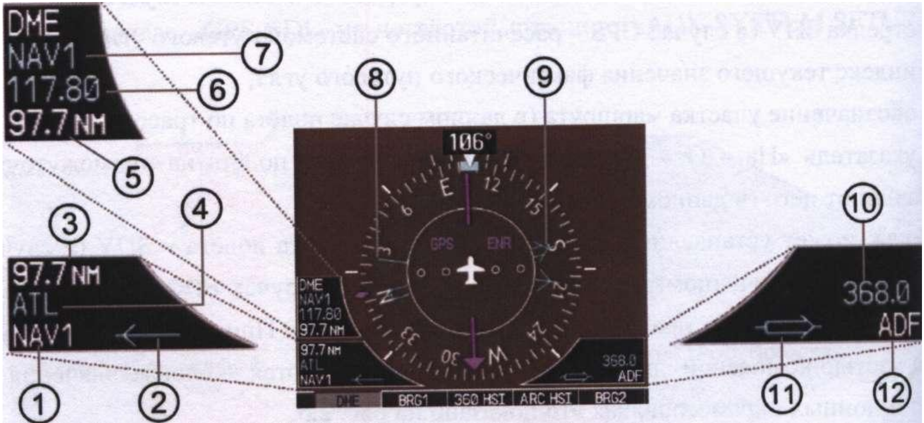
Рис. 3.14. Представление пеленгационной и дальномерной информации
