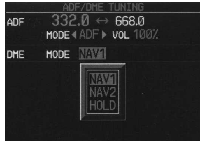
Рис. 3.2.9. Информационное окно «ADF/DME TUNING» для настройки DME
