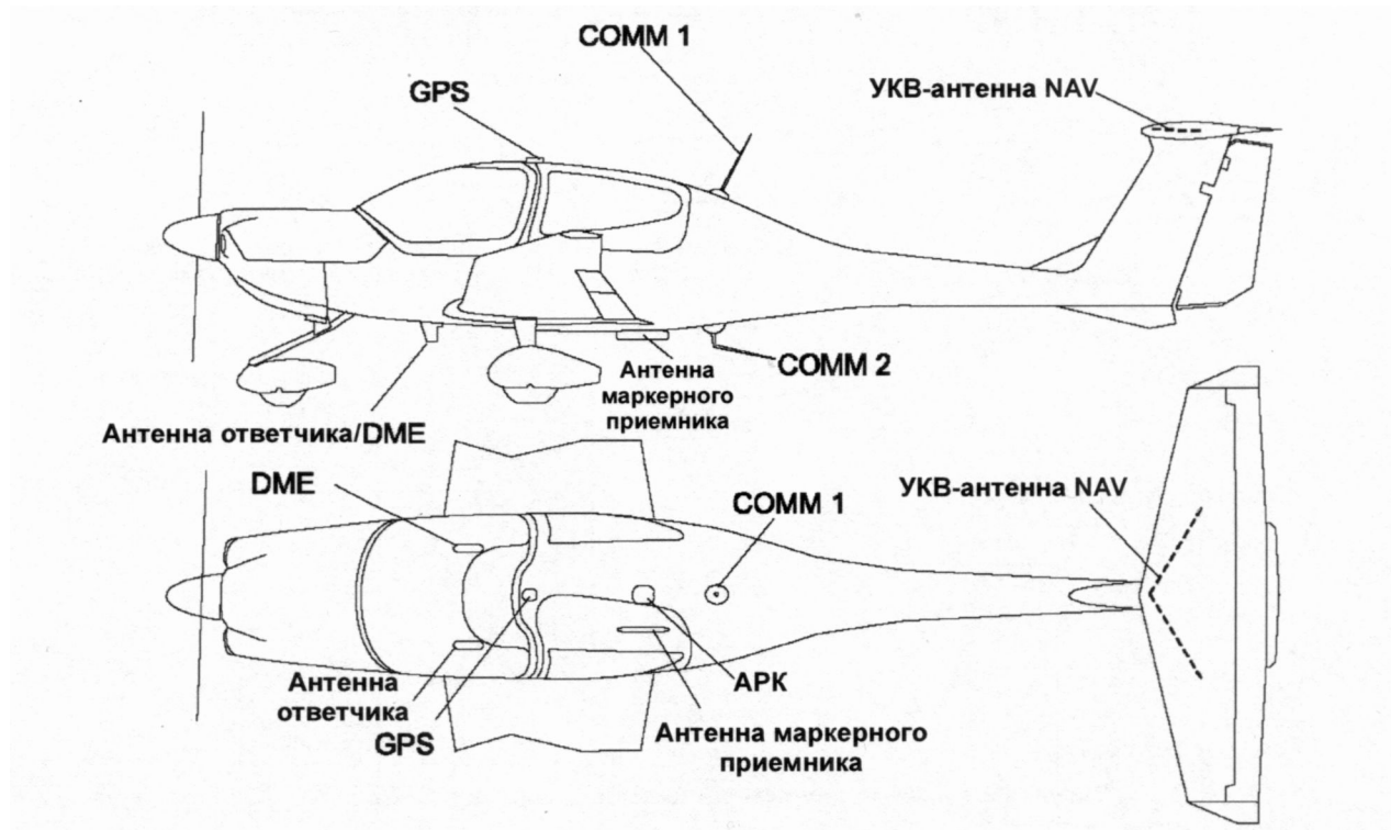
Рис 1.2. Размещение радиоантенн и датчиков приборного оборудования на ВС DA 40 (антенна маяка ELT на DA 40 размещается внутри фюзеляжа)
