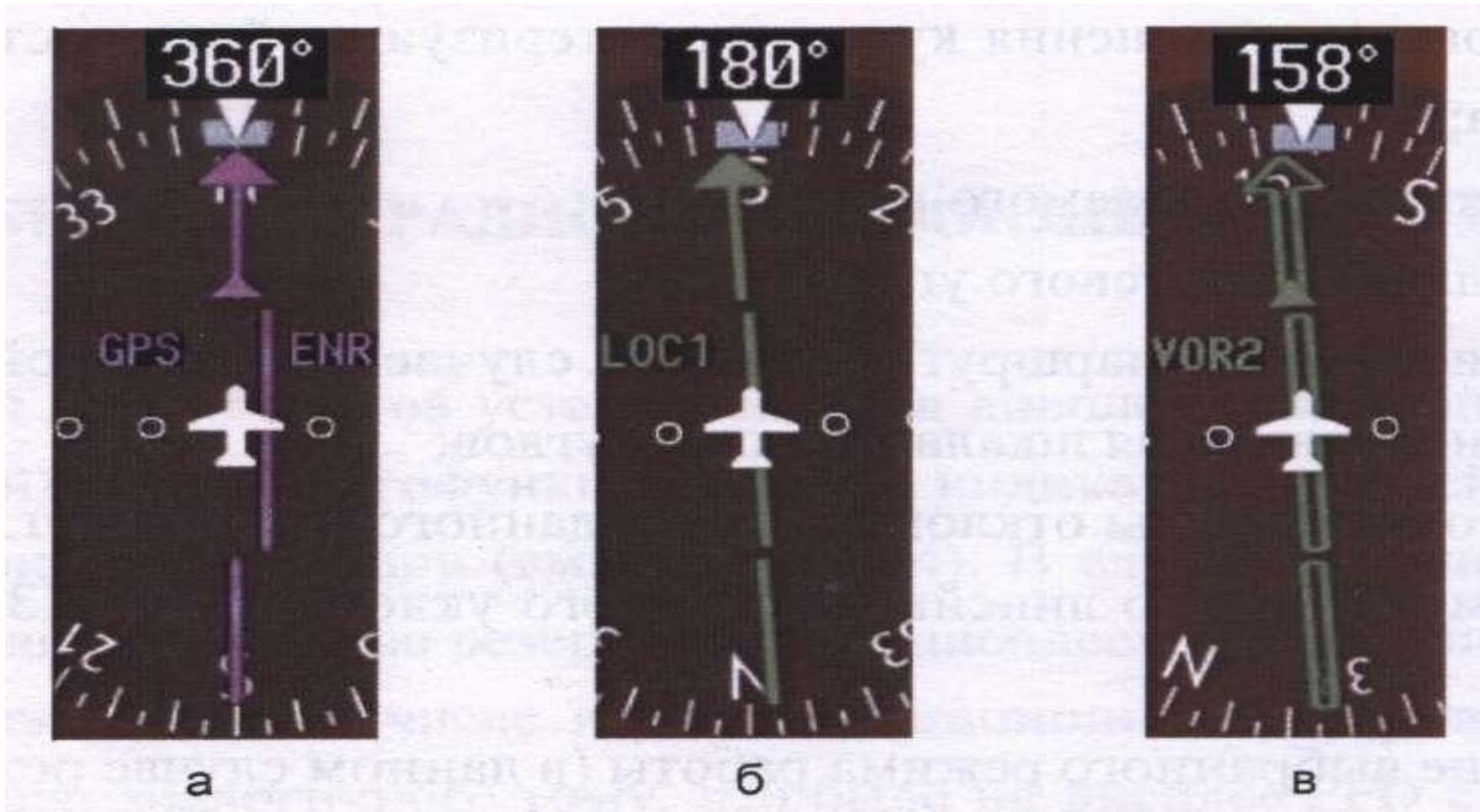
Рис. 3.5. Примеры отображения индикатора CDI в зависимости от выбранного источника радионавигационной информации для самолётовождения.
