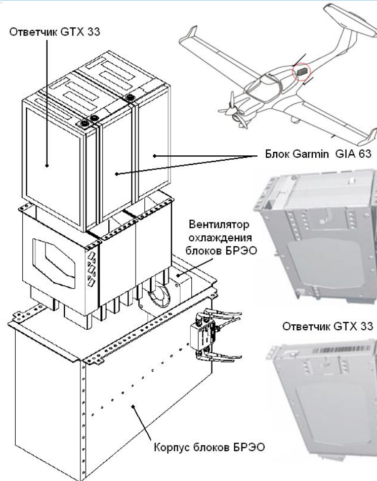
Рис. 1.10. Размещение радиоэлектронного оборудования (GIA 63, ответчик GTX 33, АРК и курсовертикаль под задним багажным отсеком)
