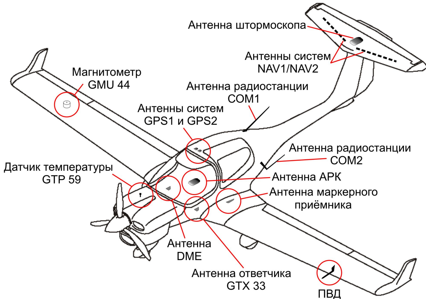
Рис 1.3. Размещение радиоантенн и датчиков приборного оборудования на ВС DA 40 (антенна маяка ELT на DA 40 размещается внутри фюзеляжа)
