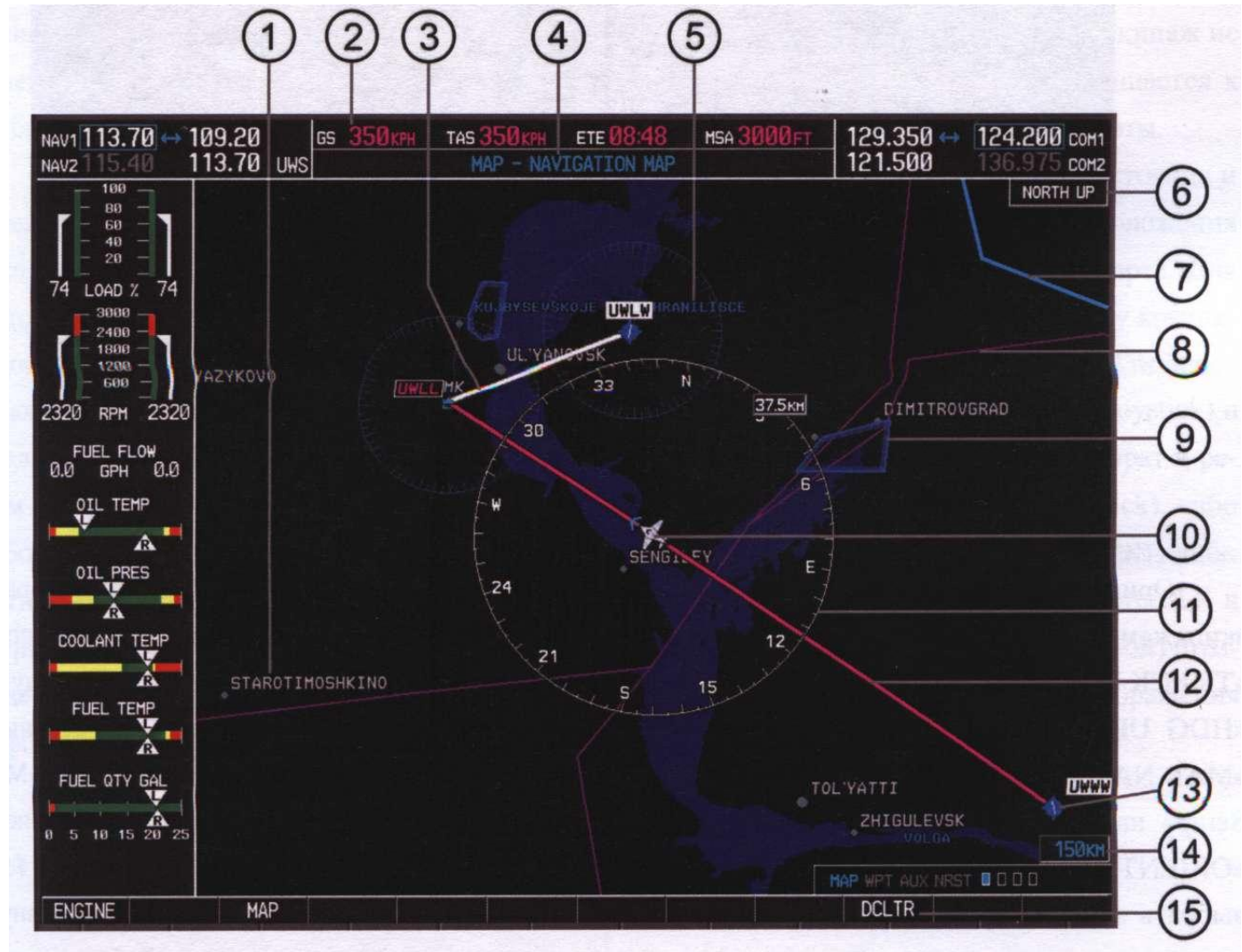
Рис. 3.3. 10. Отображение информации в режиме движущейся карты на дисплее MFD
