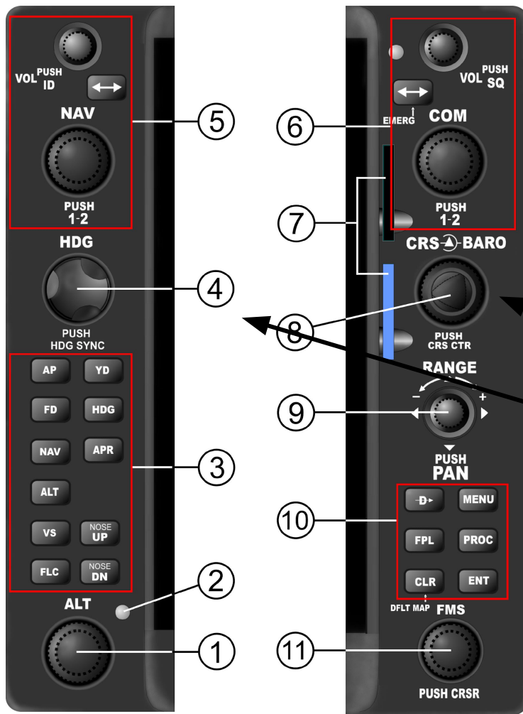
Рис.3.8.Левая и правая панель дисплеев.
