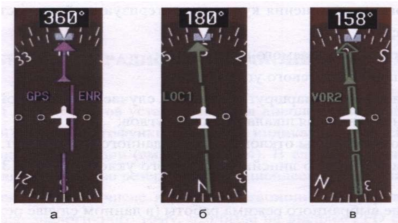
Рис.3.2.3. Примеры изображения индикатора CDI в зависимости от выбранного источника радионавигационной информации для самолётовождения
