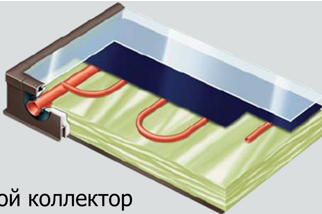
Пластинчатый коллектор
