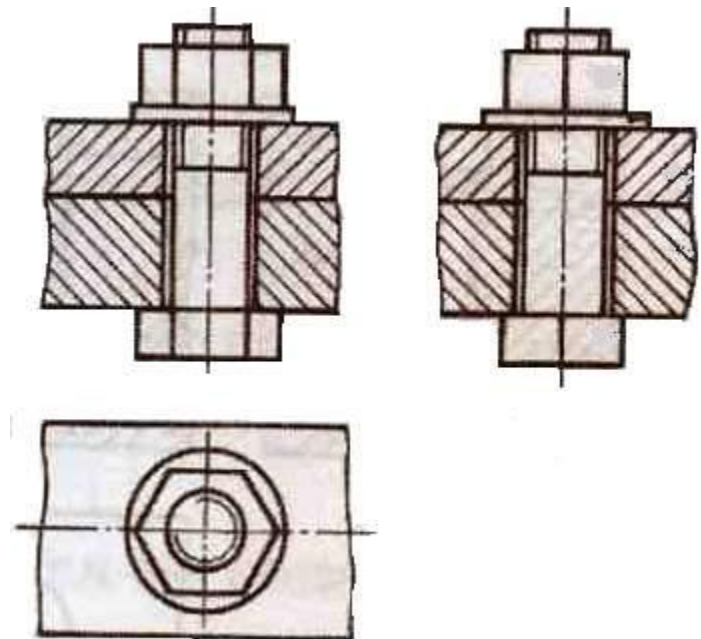
Болтовое соединение
