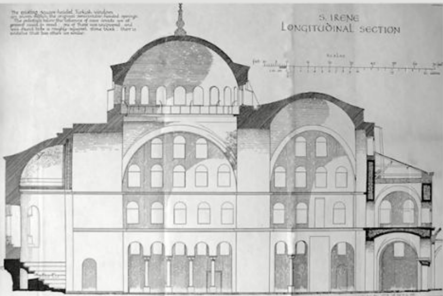
Церковь Св. Ирины (разрез). 6 — 8 вв
