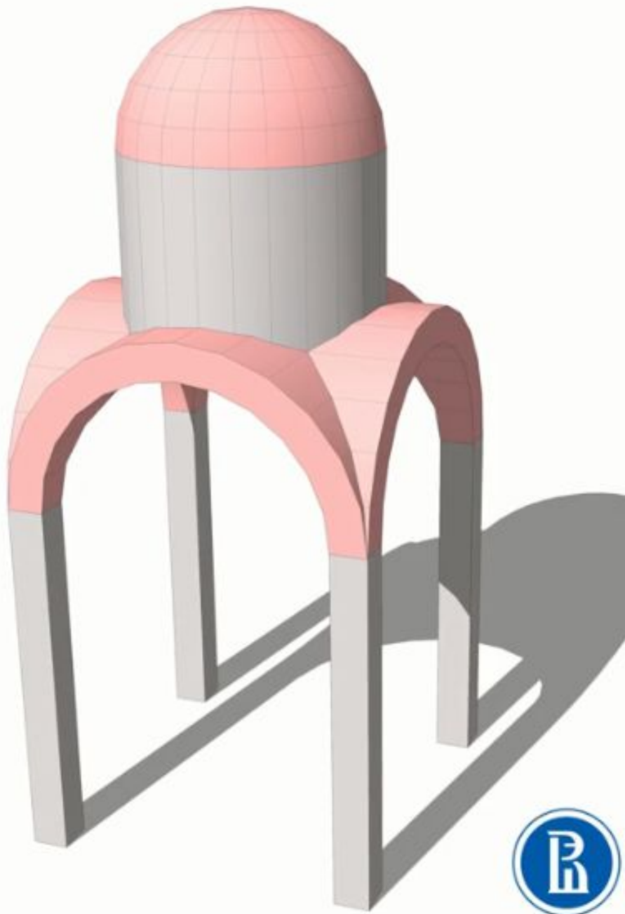
Крестово-купольная конструкция.
