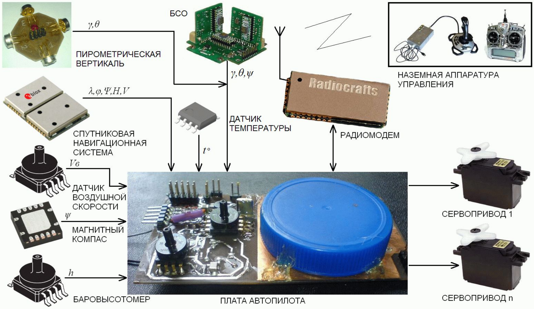
Обобщённая структурная схема авионики БПЛА "Беркучи"
