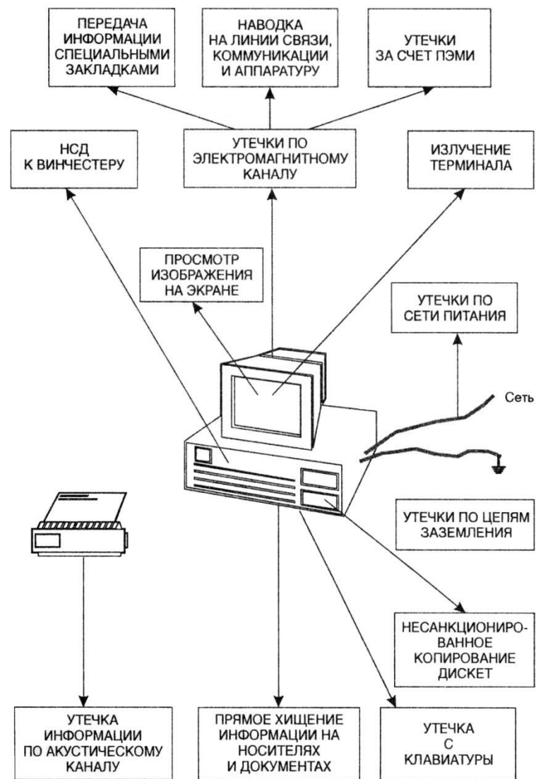
Модель каналов утечки информации и способов несанкционированного доступа ПЭВМ
