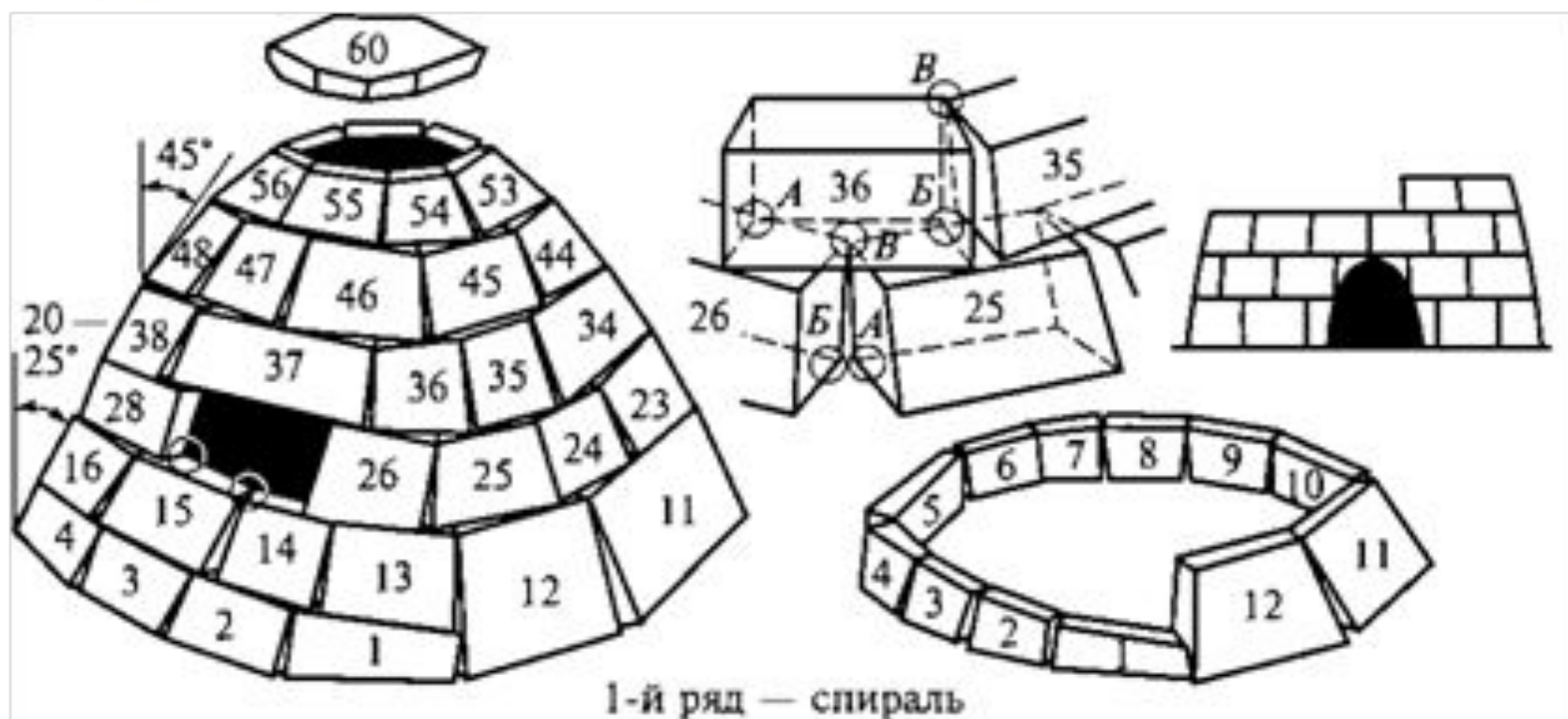
Рис. 139. Строительство иглу:
