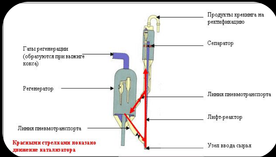
Реакторный блок каталитического крекинга по технологии ExxonMobil. В правой части - реактор, слева от него - регенератор.
