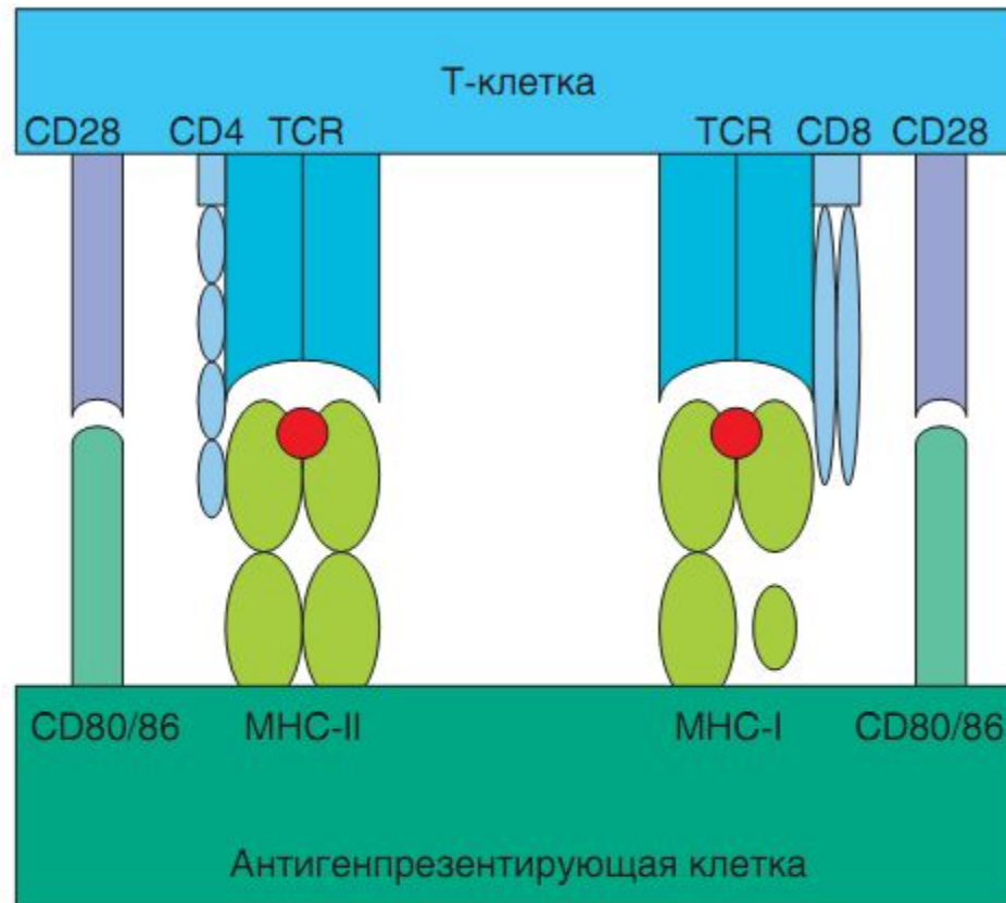
Рис. 3.88. Схема презентации антигена. Представлены все основные пары молекул, участвующие в презентации — молекулы МНС, несущие антигенный пептид, и ТСR, распознающий их с участием корецепторов (CD4, CD8), а также костимулирующие молекулы В7 (CD80/CD86) и CD28
