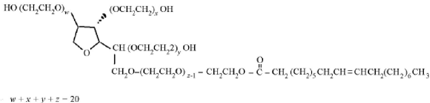
Рис. 1. Структурная формула Твина 80
