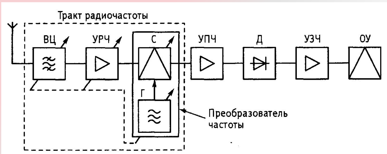
Рис. 2.20. Структурная схема супергетеродинного приемника
