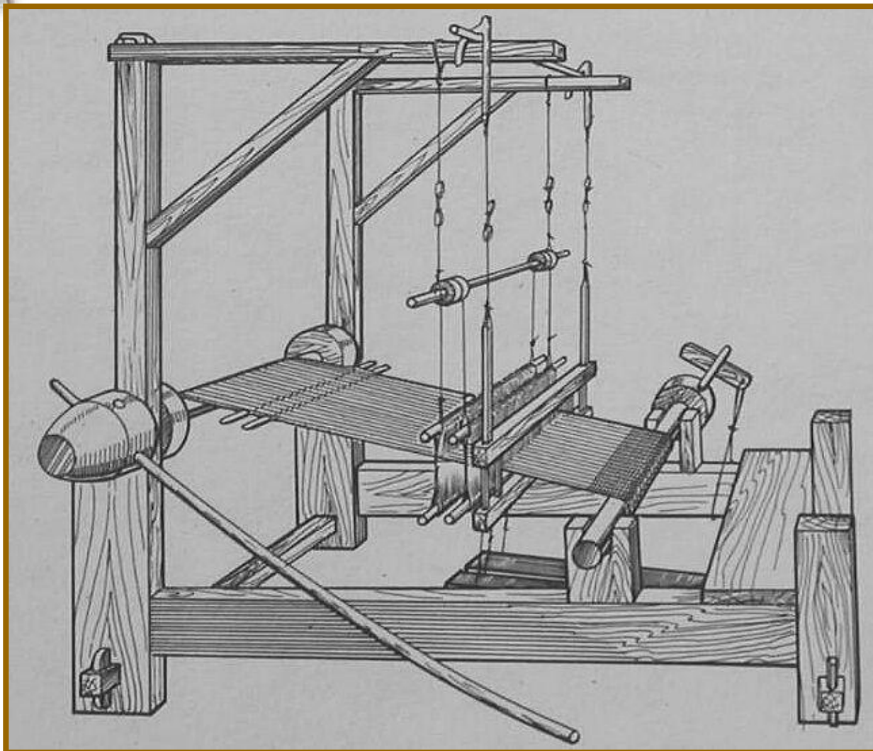
Горизонтальный ткацкий станок
