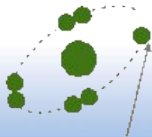
Неспаренный электрон
