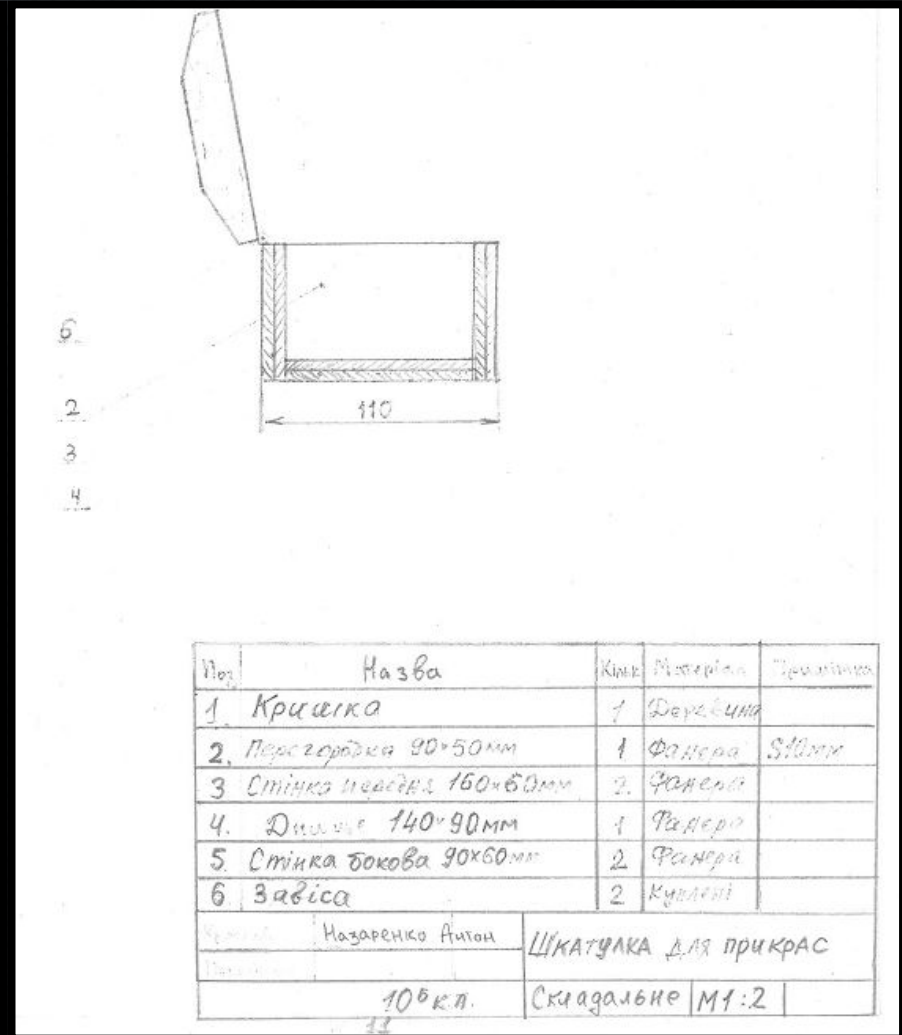
Вигляд збоку
