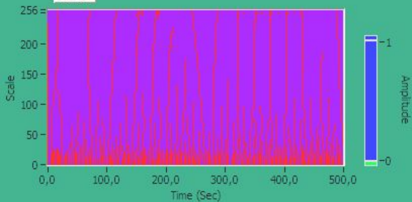
Скелет
