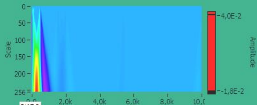
Скалограмма
