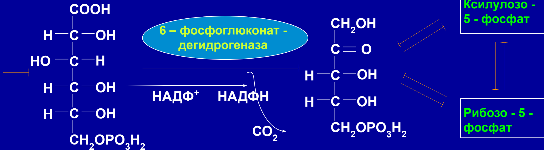
Рибозо - 5 - фосфат
