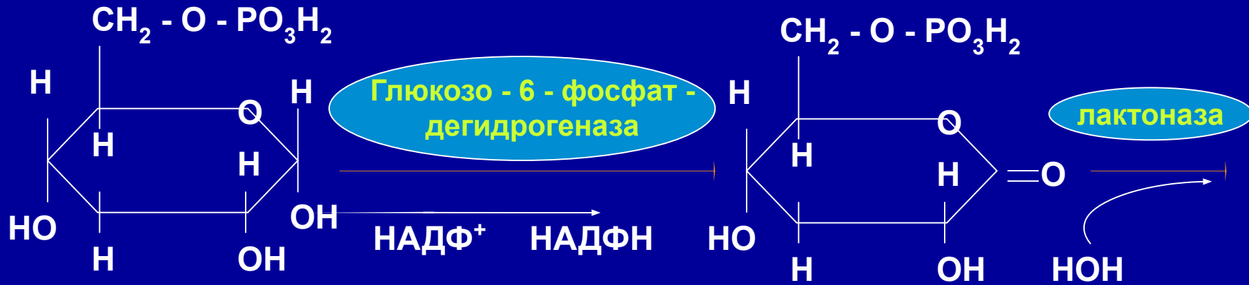
Глюкозо - 6 - фосфат
