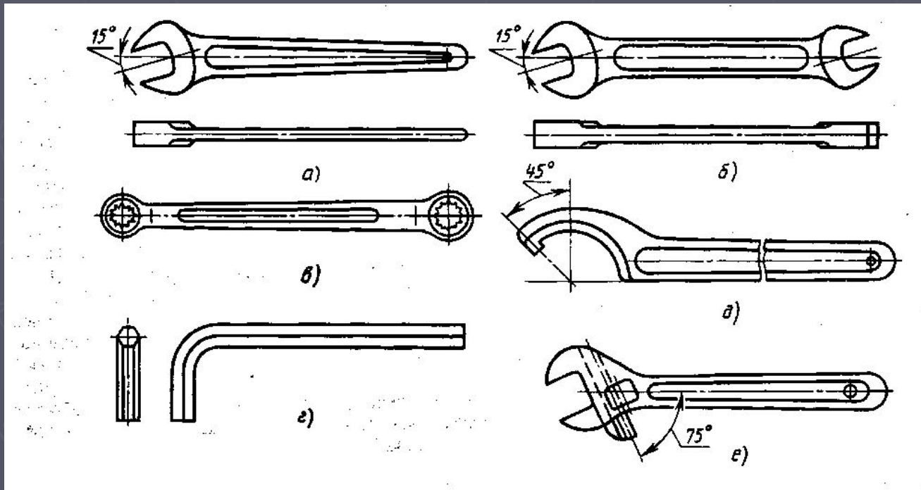
Гаечные ключи
