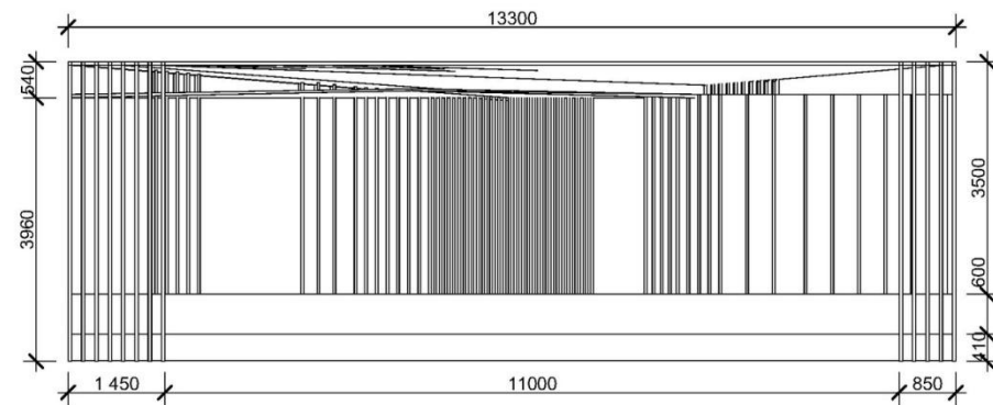
Вид спереди М 1:50
