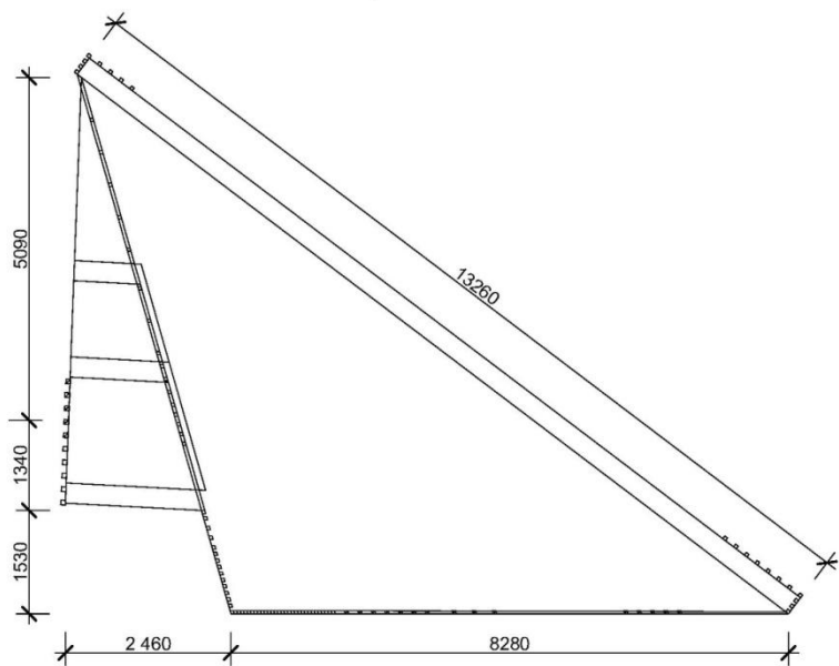
Вид сверху М 1:50
