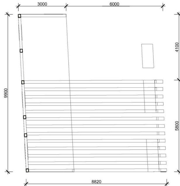
Вид сверху М 1:50
