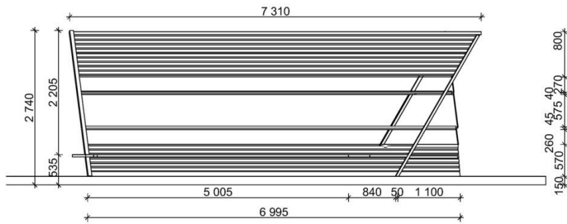
Вид сбоку М 1:50
