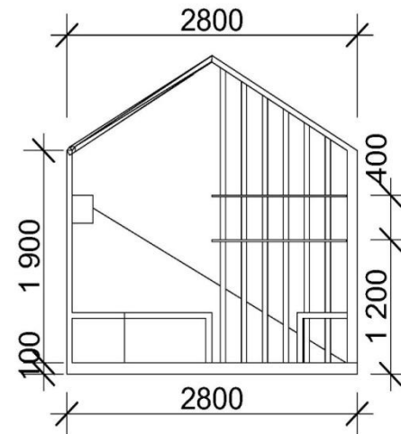
Вид спереди М 1:50
