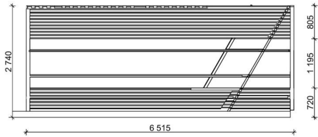
Вид сбоку М 1:50
