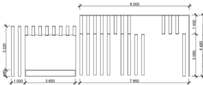
Вид сбоку М 1:50
