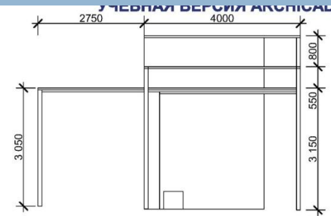
Вид спереди М 1:50
