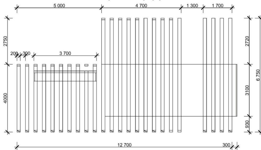
Вид сверху М 1:50
