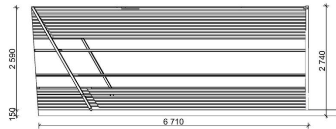
Разрез М 1:50
