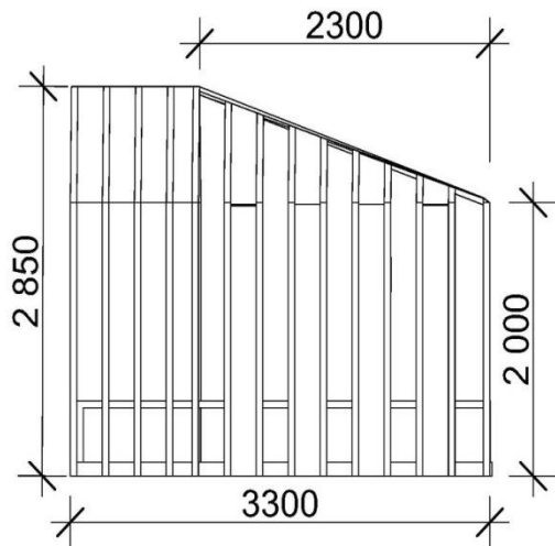
Вид сбоку М 1:50
