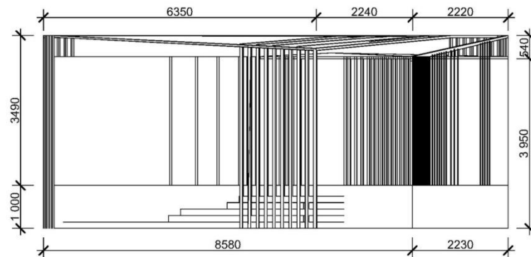
Вид сбоку М 1:50
