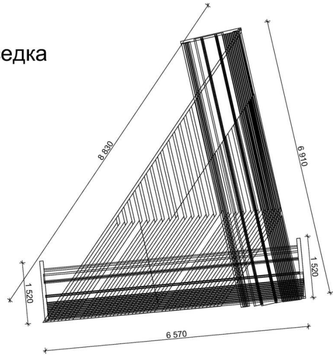
Вид сверху М 1:50
