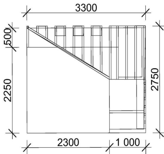
Вид сверху М 1:50
