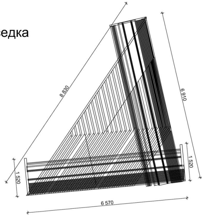
Вид сверху М 1:50
