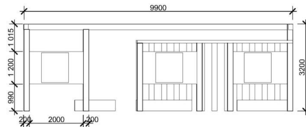
Вид сбоку М 1:50
