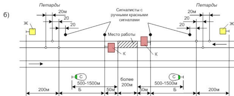
Рисунок – Схема ограждения на перегоне мест производства работ, требующих остановки поездов при фронте работ более 200 м: а – на однопутном участке; б – на одном из путей двухпутного участка; в – на обоих путях двухпутного участка
