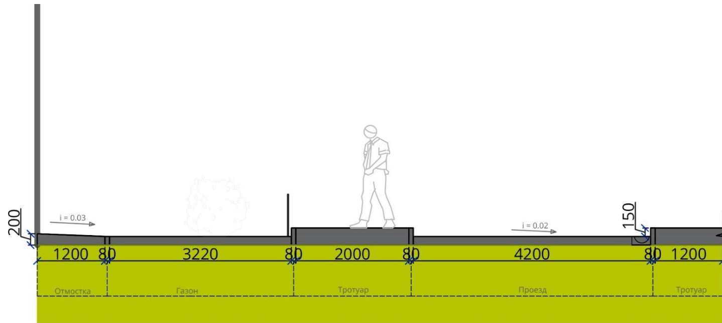
Поперечный профиль 2-2
