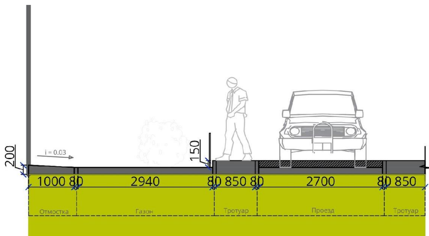
Поперечный профиль 2-2
