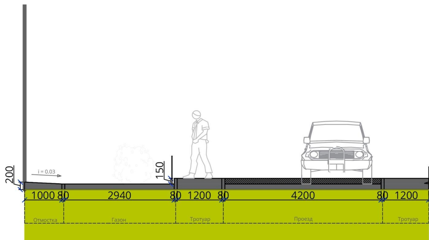
Поперечный профиль 2-2
