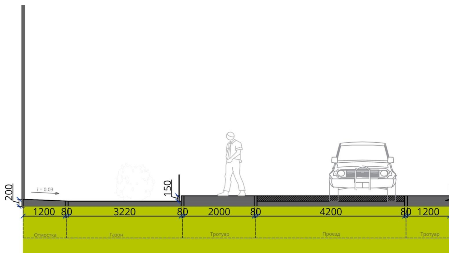
Поперечный профиль 2-2
