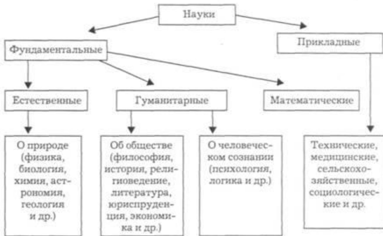
Рис. 1.2. Классификация наук
